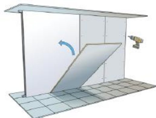
E Positionner la plaque avec le Tecsound SY sur le support et fixer mécaniquement par des vis.
